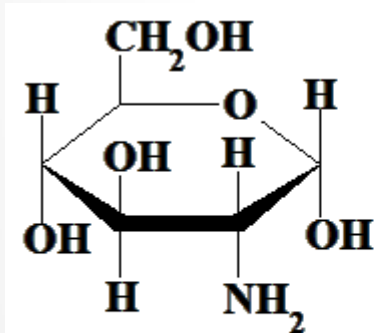
GLUKOSAMIN
