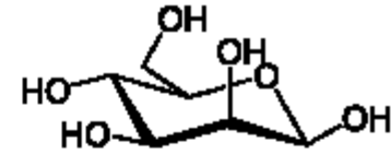
\beta -D-Man
