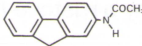
2-Acetaminofluoren
