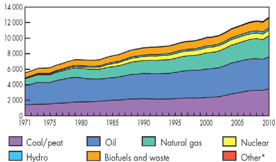
Obr. 15 Celková světová výroba energie 1971-2010 dle zdroje. 131 * zahrnuje geotermální, solární, větrnou E, atd.
