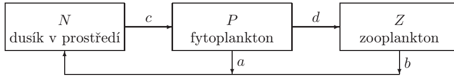
Obrázek 10.1: Schéma koloběhu dusíku
