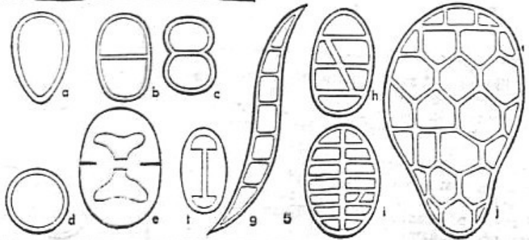
Stavba stélky a plodnic lišejníků: 1 svislý řez heteromerickou stélkou, a kůra, b stélkové řasy, c dřeň, d rhizidy; 2 různé druhy sorálů, a rtovitý, b jazykovitý, c kápovitý; 3 svislý řez peritheciem, a vřeska s výtrusy, b kůra, c stélkové řasy, d dřeň; 4 svislý řez apotheciem, a thecium, b hypothecium, c epithecium, e stélkový okraj apothecia, f viasní okraj apothecia (excipulum), g kůra, h stélkové řasy, i dřeň; 5 různé druhy výtrusů, a, d jednobuněčné, b, c, e, f dvoubuněčné, g mnohobuněčné s příčnými přehrádkami, h, i mnohobuněčné s příčnými a podélnými přehrádkami
