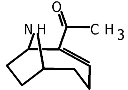
Anatoxin-a
