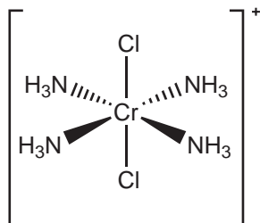
trans -dichloro-tetramminochromitan
