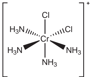
cis -dichloro-tetramminochromitan
