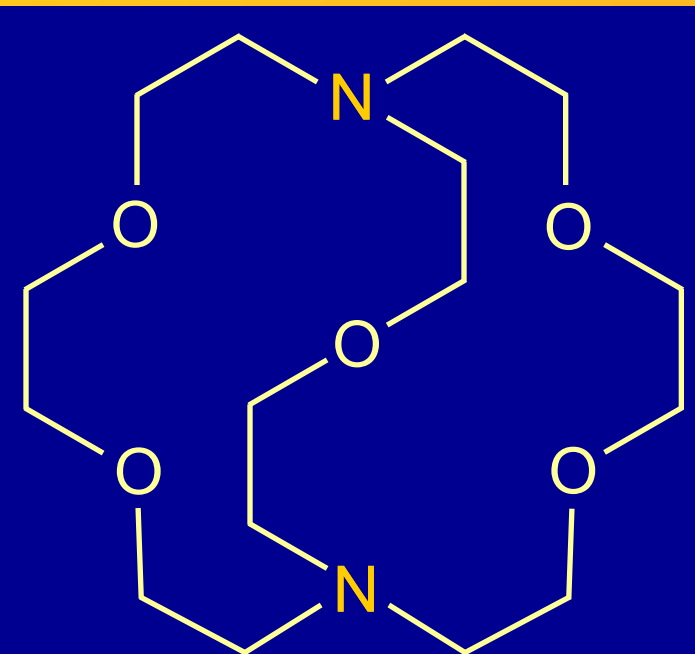
2,2,1-kryptand
