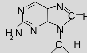
9-ribose-2-aminopurine
