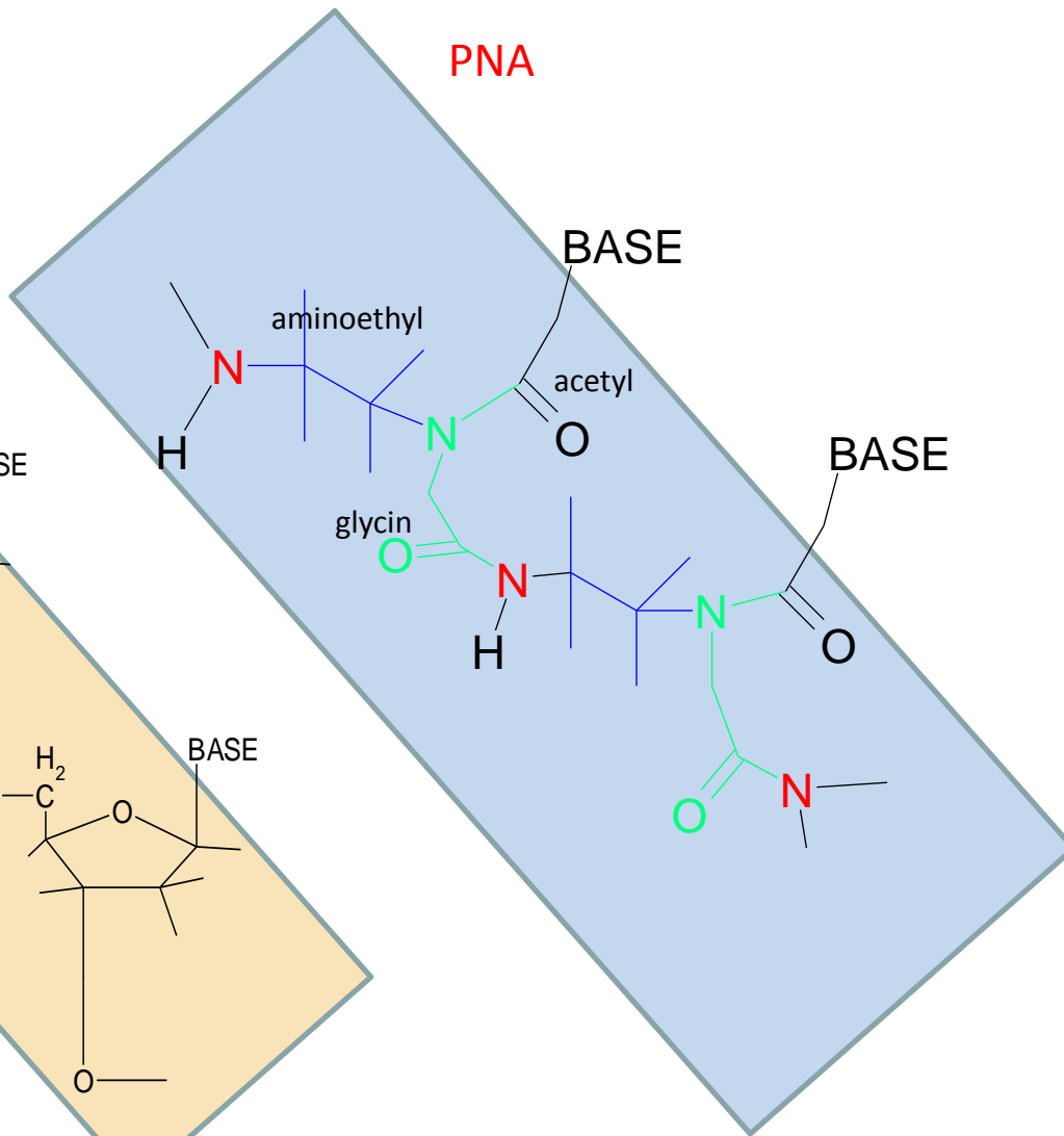
POLYAMINOETHYLGLYCIN
