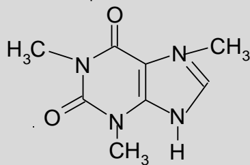
caffeine
