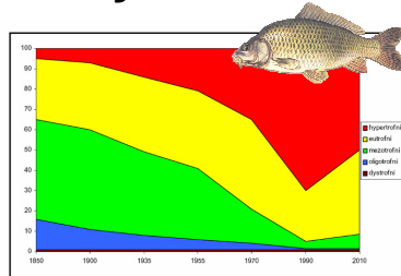
Obr. 4: Změny v podílu rybníků s různou trofíí vody od poloviny 19. století.
