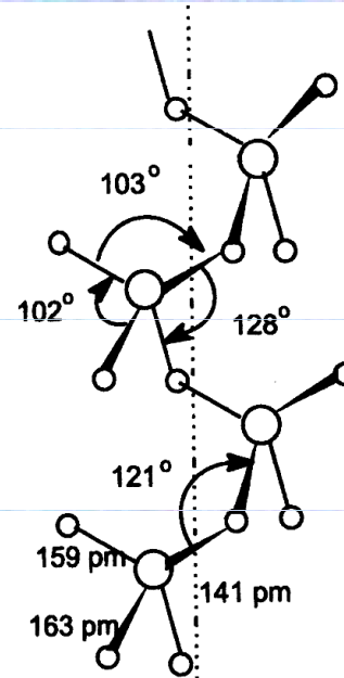
polymer SO 3
