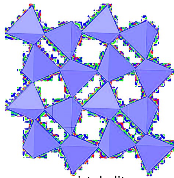
cristobalit
