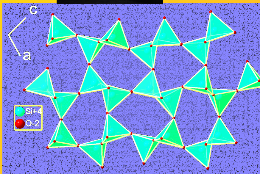
tridymit
