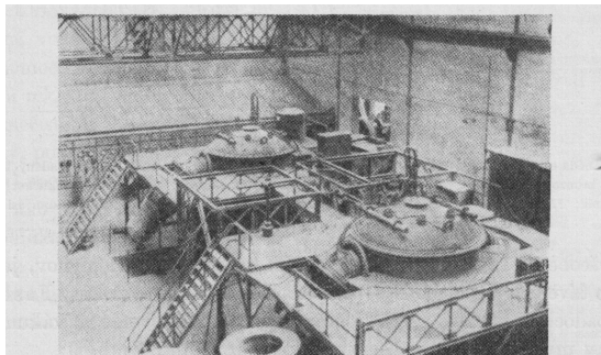
Obr. 9,2-6. Vákuová taviaca pec pre vsádzku 4 t s vákuovotesne nasadenými kokilami (Rohn; výroba: Heraeus Vacuumschmelze).
