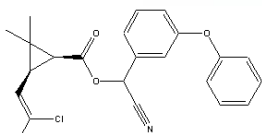
Cypermethrin
