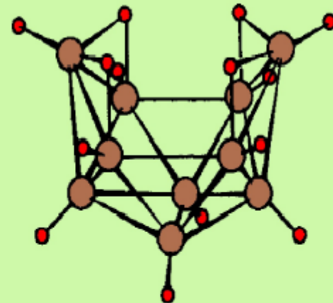
dekaboran(14) B_{10}H_{14}
