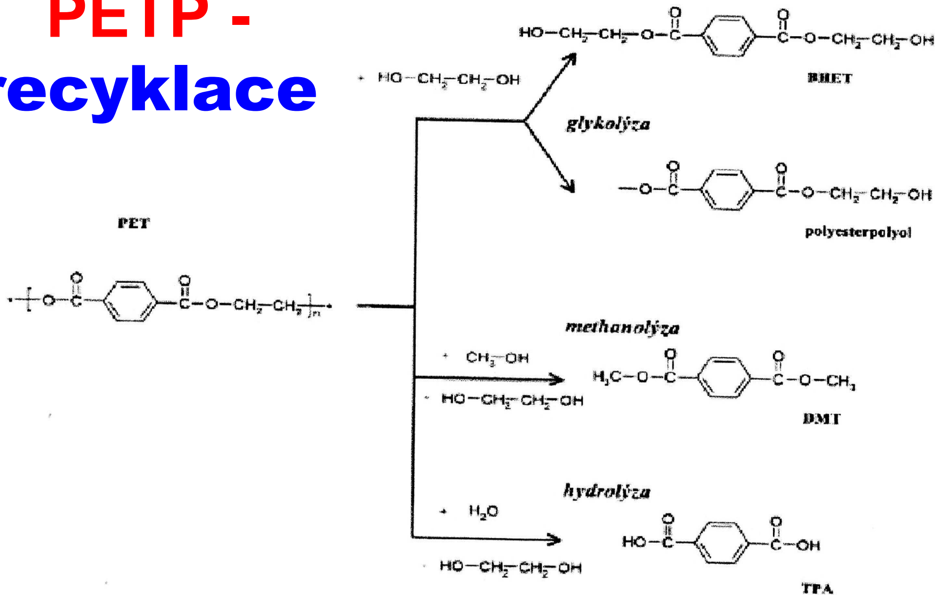
Obr. 8 Různé způsoby solvolýzy PET.
