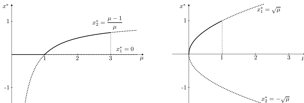
Obrázek 5.2: Rovnovážné body logistické rovnice (5.13) (vlevo) a rovnice (5.14) (vpravo) v závislosti na hodnotách parametru \mu . Asymptoticky stabilní rovnovážný bod je znázorněn plnou čarou, nestabilní tečkovanou čarou.
