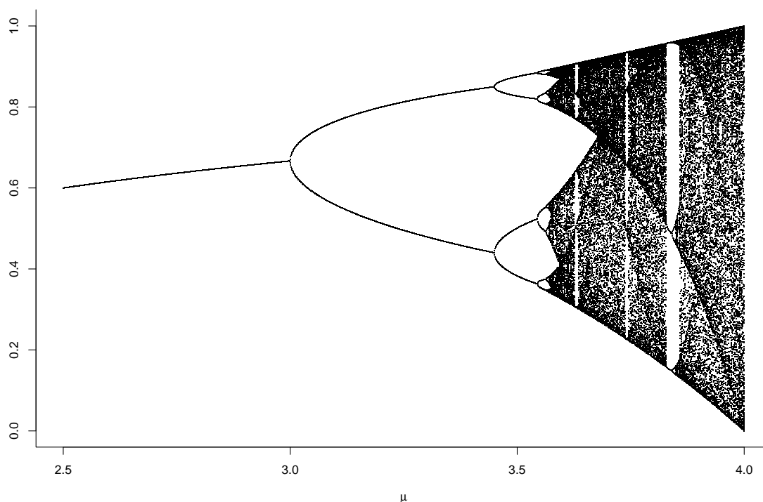
Obrázek 5.3: Bifurkační diagram logistické rovnice (5.13)
