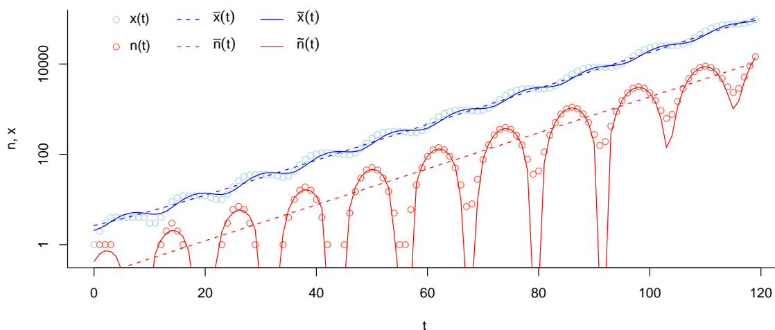
Obrázek 7.2: Upravený model „rozmnožování lidského rodu“ (7.15). Na svislé ose je logaritmické měřítko. Symboly označují: x(t) , n(t) — hodnoty počítané z rekurentních vztahů (7.15), \bar{x}(t) , \bar{n}(t) — první aproximace řešení (7.17) využívající pouze dominantní charakteristický kořen \lambda_1 (trend), \tilde{x}(t) , \tilde{n}(t) — druhá aproximace řešení (7.19) využívající charakteristické kořeny \lambda_{2,3} s druhým největším modulem. Při výpočtu byly použity hodnoty \alpha \doteq 0,194708013278096 , \bar{x}_0 \doteq 2,6514514395602 , \beta \doteq 0,231889637997667 , \gamma \doteq 0,352845633763305 , \tilde{x}_0 \doteq 2,07362768022334 .
