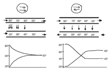
Obr. 14.9: Srovnání stejnosměrné a protiproudé výměny na příkladě teplot. Zatímco při stejnosměrné gradient klesá, až se výsledná teplota ustálí na průměru, při protiproudé výměně je gradient po celé délce konstantní a výměna tepla je účinnější.
