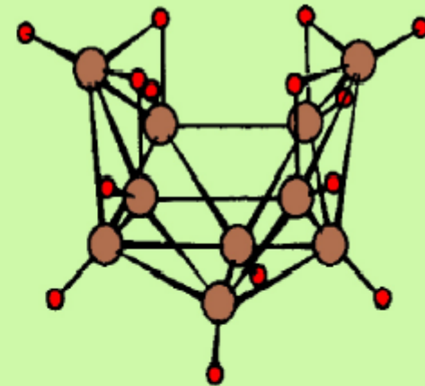
dekaboran(14) B_{10}H_{14}
