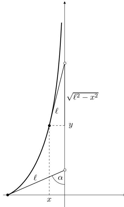
Obrázek 5.1: Traktrisa
