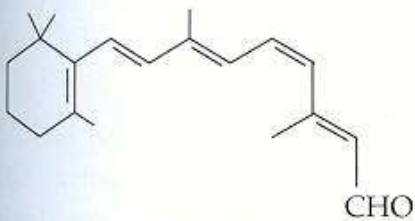
Retinal (11-cis)
