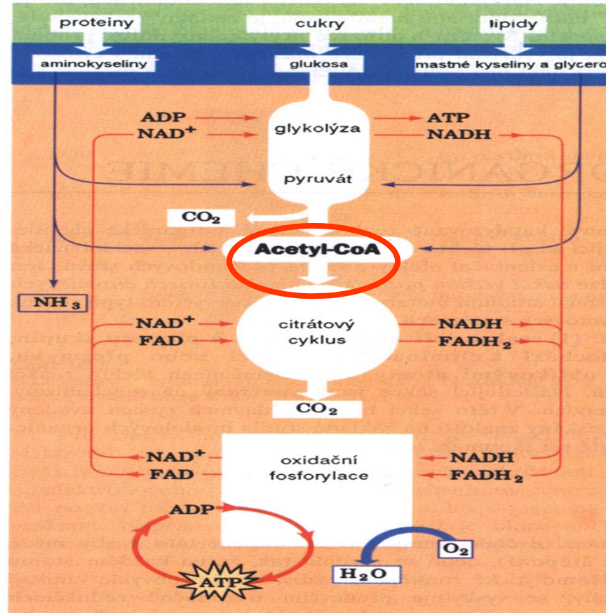
Obr. 15-3 Složité metabolity, jako jsou sacharidy, lipidy a proteiny, jsou nejprve degradovány na své monomerní jednotky, hlavně glukosu, mastné kyseliny a aminokyseliny, a dále na společný meziprodukt – acetyl-CoA. Acetylová skupina je poté oxidována kyslíkem na oxid uhličitý přes citrátový cyklus za současné redukce \text{NAD}^+ a \text{FAD} . Reoxidace těchto koenzymů přes řetězec přenosu elektronů a oxidační fosforylaci vede ke vzniku vody a ATP.
