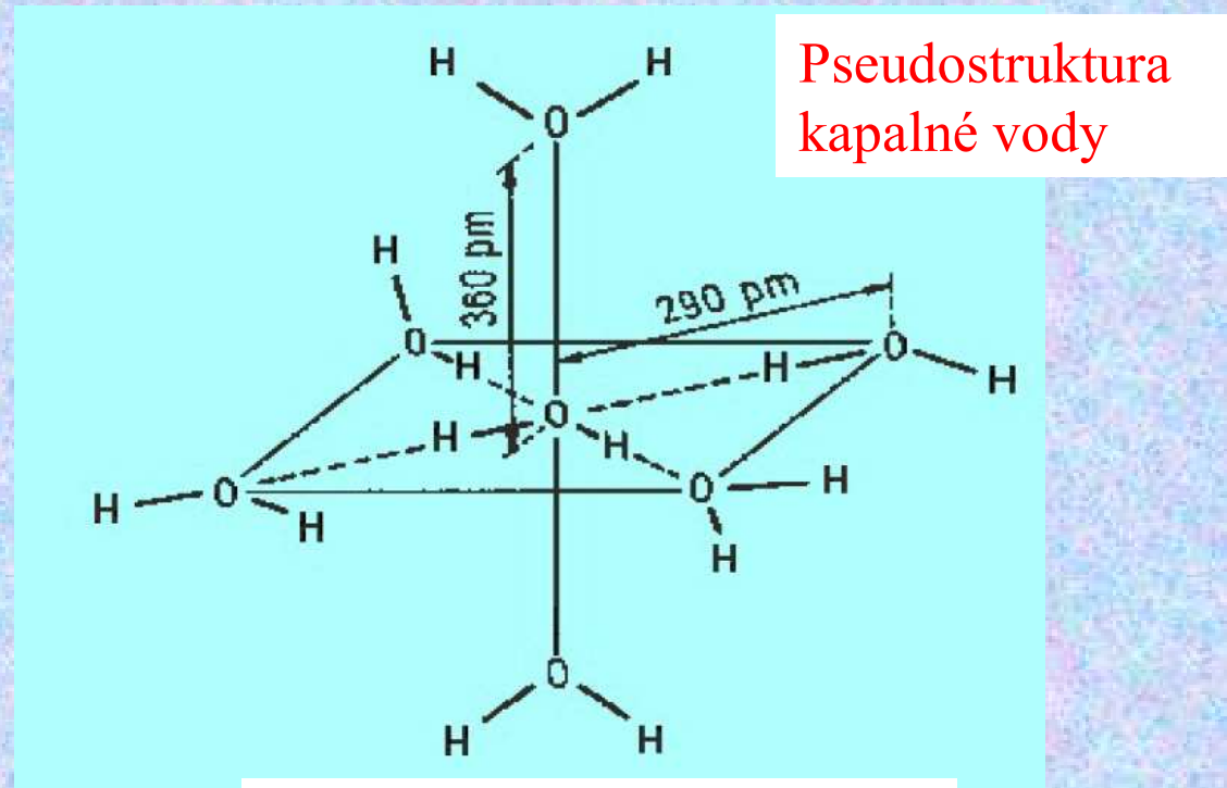
tetragonální soustava
