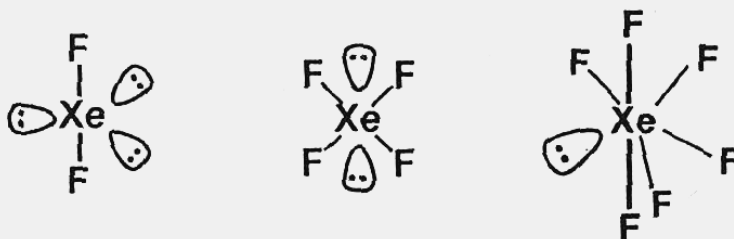
Obr.č. 10.1. Fluoridy xenonu
