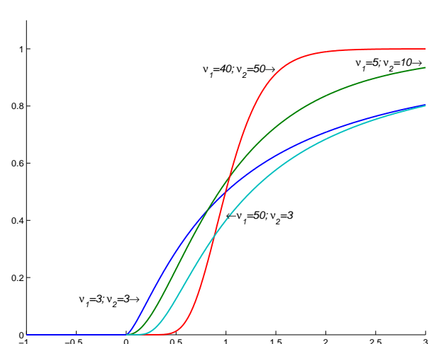
Grafy distribučních funkcí Fisherova–Snedecorova F rozdělení
