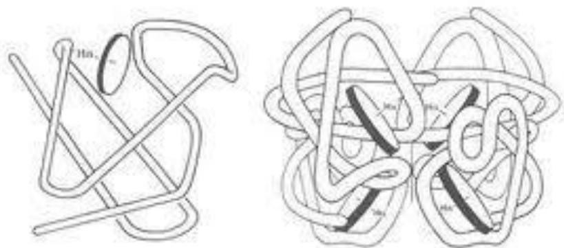
Haemoglobin
