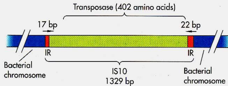
Struktura inzerční sekvence IS10
