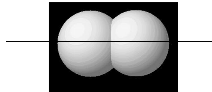
Lineární molekuly
