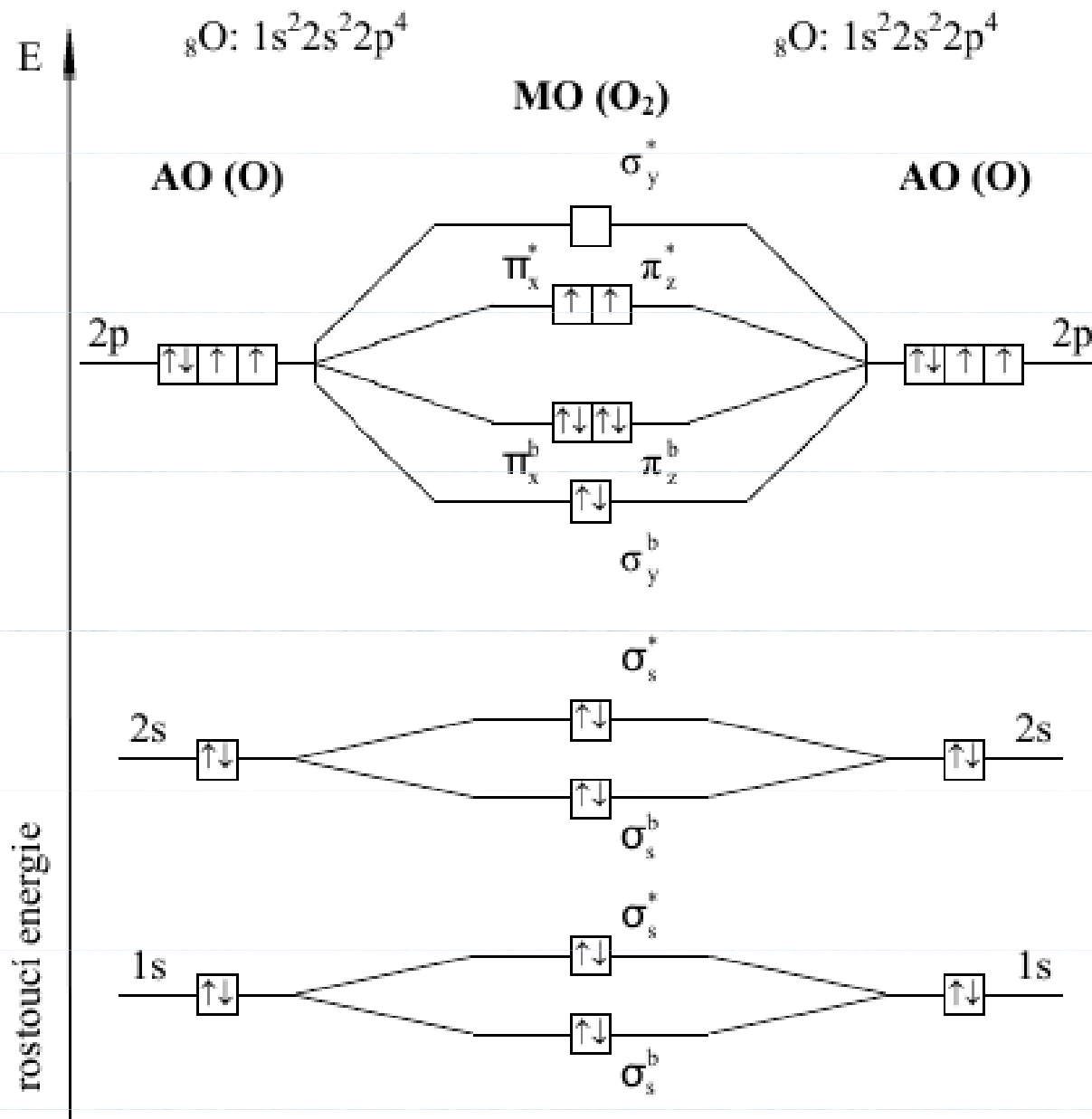
Obr. 10-10: Diagram MO pro stabilnější formu O_2 (tripletový stav).
