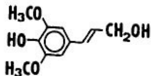
sinapinalkohol
