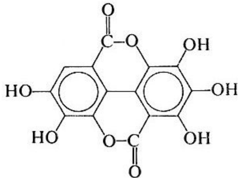
kyselina elagová
