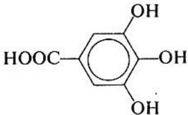
kyselina galová
