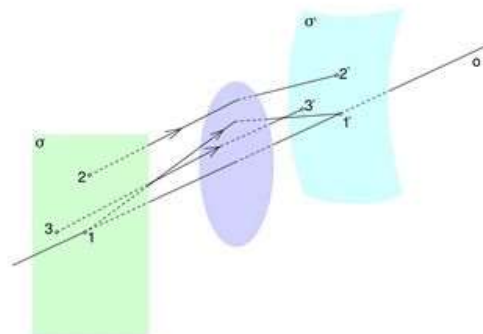
Zklenutí pole
