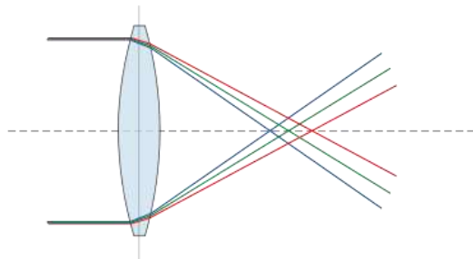
Chromatická aberace
