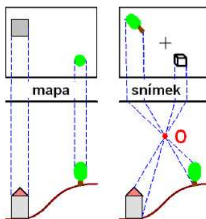
Pravouhlé promítání
