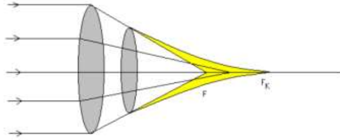
Sférická vada
