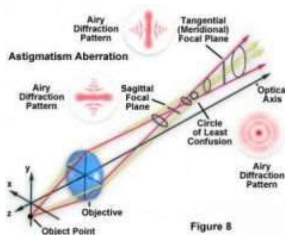
Astigmatická vada
