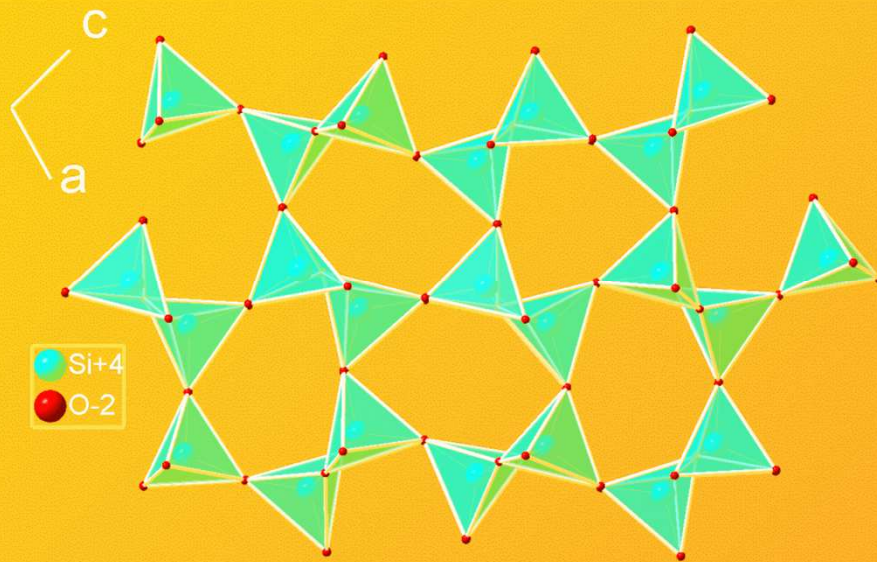
tridymit
