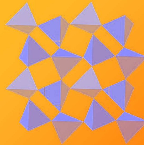
cristobalit
