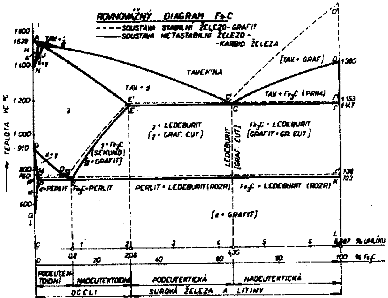
Obr. 31.2 Rovnovážený diagram Fe-C.
