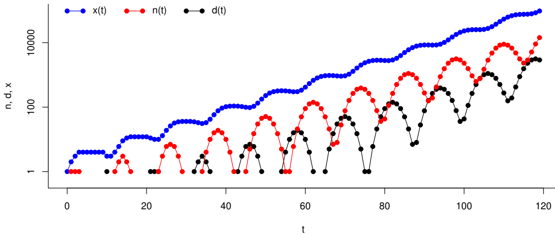
Obrázek 6.1: Model „rozmnožování lidského rodu“ (6.14). Na svislé ose je logaritmické měřítko. Symbols označují: x(t) — počet žijících párů v čase t , tj. 2t let od počátku, n(t) — počet narození v čase t , d(t) — počet úmrtí v čase t .
