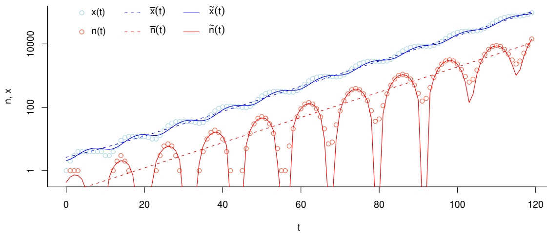
Obrázek 6.2: Upravený model „rozmnožování lidského rodu“ (6.15). Na svislé ose je logaritmičké měřítko. Symboly označují: x(t) , n(t) — hodnoty počítané z rekurentních vztahů (6.15), \bar{x}(t) , \bar{n}(t) — první aproximace řešení (6.17) využívající pouze dominantní charakteristický kořen \lambda_1 (trend), \tilde{x}(t) , \tilde{n}(t) — druhá aproximace řešení (6.19) využívající charakteristické kořeny \lambda_{2,3} s druhým největším modulem. Při výpočtu byly použity hodnoty \alpha \doteq 0,194708013278096 , \bar{x}_0 \doteq 2,6514514395602 , \beta \doteq 0,231889637997667 , \gamma \doteq 0,352845633763305 , \tilde{x}_0 \doteq 2,07362768022334 .
