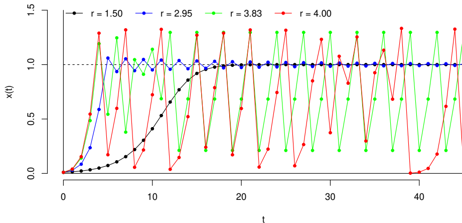
Obrázek 1.2: Řešení logistické rovnice x(t+1) = x(t)(r - (r-1)x(t)) s počáteční hodnotou x(0) = 0,01 pro několik hodnot parametru r . Pro r = 1,5 je řešením rostoucí posloupnost s limitou 1 (rovnovážná velikost populace), pro r = 2,95 řešení konverguje k hodnotě 1 s tlumenými oscilacemi, pro r = 3,83 řešení pro dostatečně velké hodnoty času t (zhruba od t = 15 ) skoro pravidelně osciluje kolem hodnoty 1 s periodou 3, pro r = 4 nelze žádnou pravidelnost řešení vysledovat.
