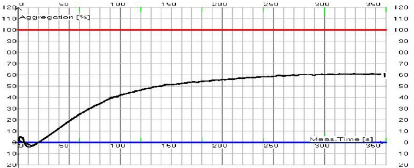
ADP 5 \mu\text{M} desagregace – křivka č. 10
