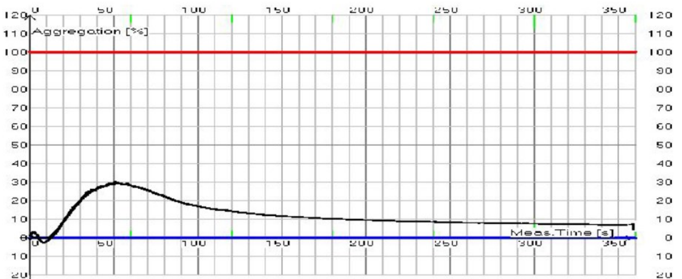
ADP 5 \mu\text{M} desagregace – křivka č. 10
