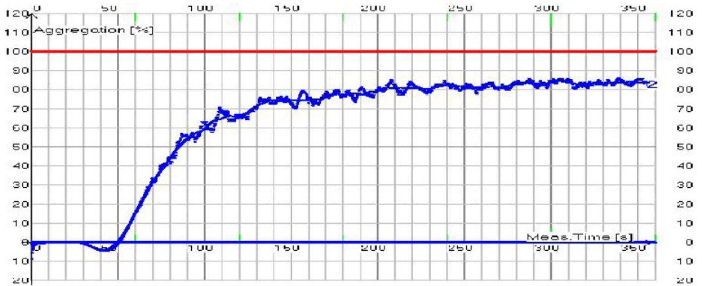
Kolagen 2 \mu\text{g}/\text{ml} – křivka č. 10
