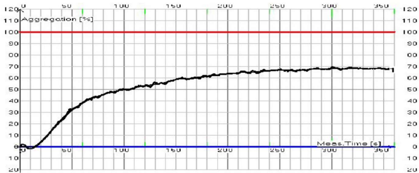
ADP 5 µM desagregace – křivka č. 6
