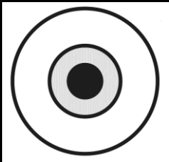
protostélé
