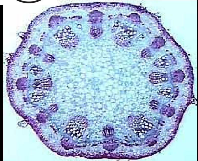
eustélé
