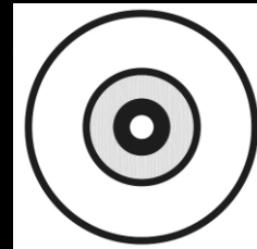
ektofloické sifonostélé
