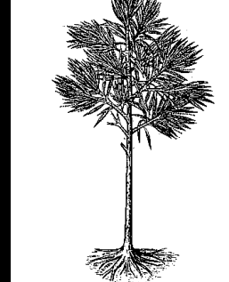
Cordaitophyta kordaity †
