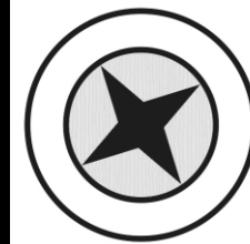
aktinostélé
