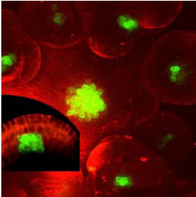
WUS::ALCR alcaA::GFP
