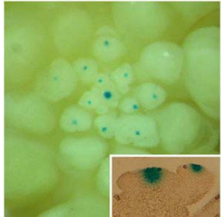
CLV3::ALCR alcaA::GUS
