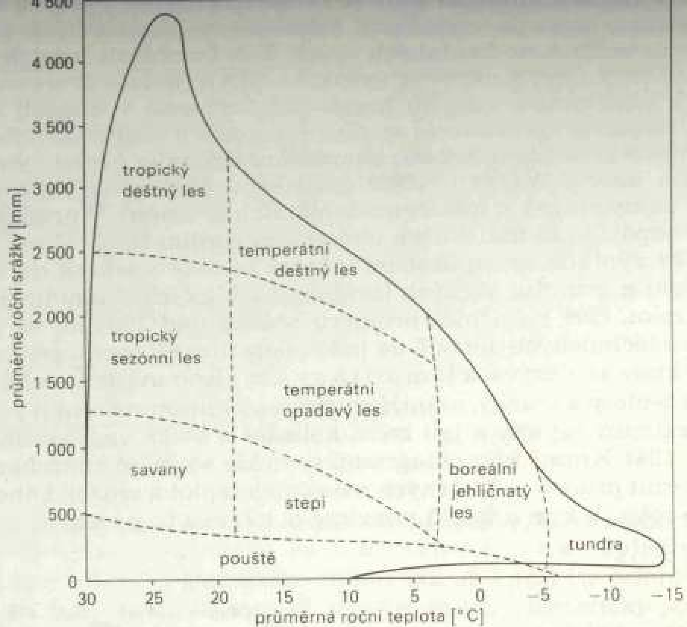
122/ Rozšíření biotů v závislosti na průměrném úhrnu ročních srážek a průměrných ročních teplotách (podle WHITTAKERA 1973)
