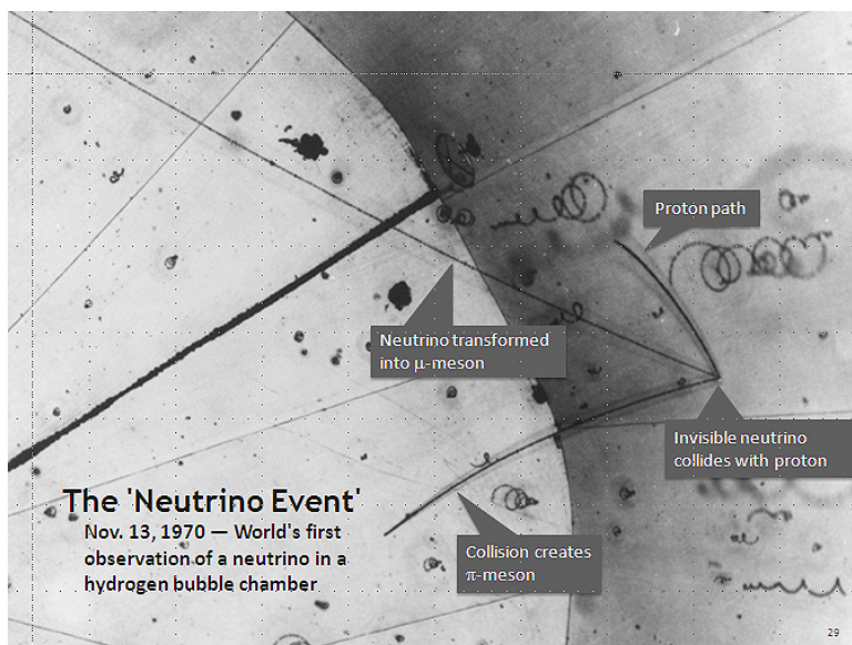
Obrázek 7.7: První detekce neutrino 13. listopadu 1970. Neutrino se srazilo s protonem v atomu vodíku. Srážka se objevila v bodě, odkud vychází tři trajektorie (na obrázku vpravo). Zdroj: Argonne National Laboratory
