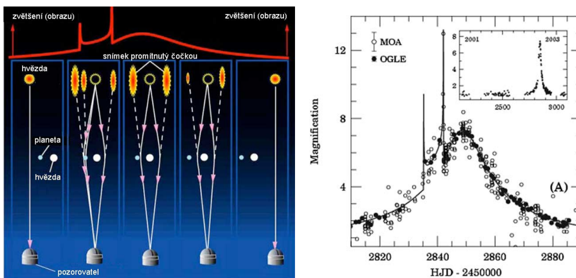
Obrázek 13.6: Vlevo: Ilustrace metody gravitační mikročočky v detekci exoplanet. Převzato z http://astronomia.zcu.cz . Vpravo: Pozorování planety gravitační mikročočkou v projektu OGLE (Bond et al., 2004). Vložený obrázek ukazuje všechna měření hvězdy z projektu OGLE v letech 2001 až 2003. Hlavní obrázek ukazuje bližší pohled na data z roku 2003 ze dvou projektů OGLE a MOA.
