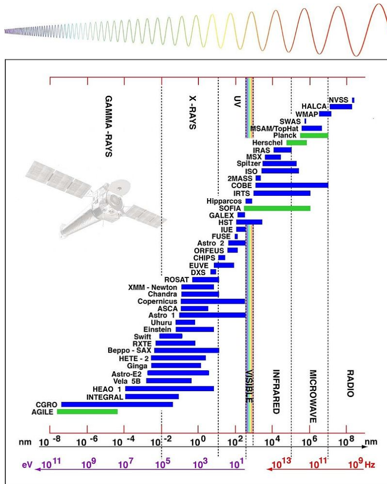
Obrázek 10.22: Významné astronomické observatoře v kosmu do r. 2005. Zdroj: https://www.wikiwand.com
