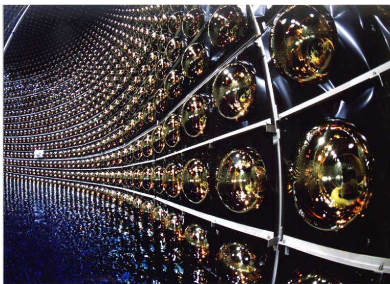
Obrázek 7.8: Skleněné baňky s fotonásobiči v detektoru neutrino Super-Kamiokande. Zdroj: Japan Radio Glass Co.,Ltd.
