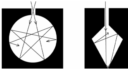
Obrázek 7.16: Model absolutně černého tělesa. Převzato z Pokorný (2006).
