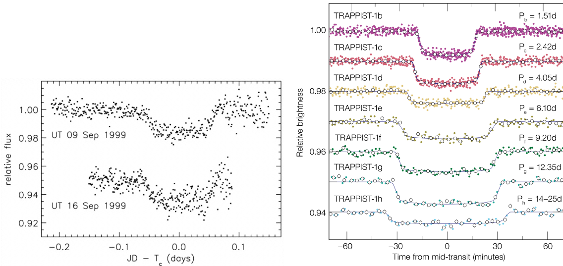
Obrázek 13.10: Vlevo: První zaznamenané tranzity exoplanety HD 209458 b. Zdroj: Charbonneau et al. (2000). Vpravo: Transitní planet v unikátní soustavě TRAPPIST-1. Zdroj: https://www.eso.org/public/news/eso1706/
