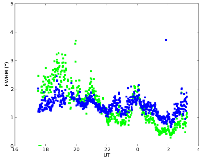
Obrázek 5.17: Změna vlastností atmosféry nad pozorovacím stanovištěm může působit i poměrně rychlé změny v seeingu. Na obrázku je průběh seeingu během noci 9./10. března 2012 na observatoři SAAO v Sutherlandu v Jižní Africe. Barevně jsou odlišeny různé metody měření.
