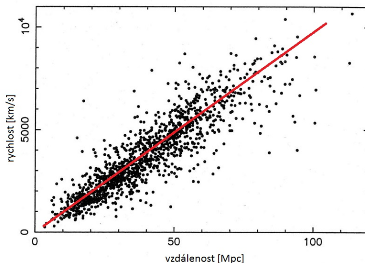
Obrázek 2.8: Závislost rychlosti vzdalování galaxií na jejich vzdálenosti od nás pro 1355 galaxií. Proložena přímkou značí Hubbleův zákon. Převzato z Liddle (2005).
