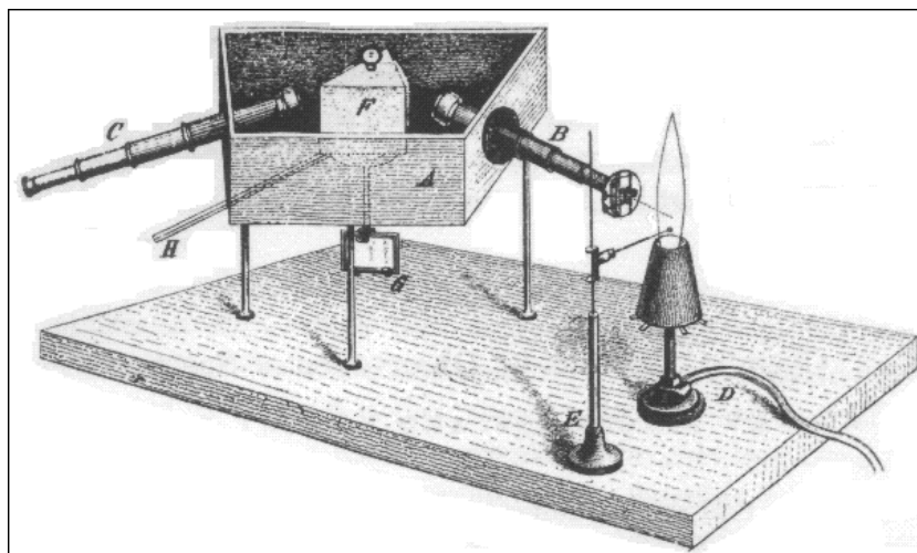
Obrázek 8.3: Spektroskop Kirchhoffa a Bunsena, A dřevěný box, B,C dalekohledy, na konci B je štěrba, D je Bunsenův hořák, E stojánek s platinovým drátkem ve spirále, kde byl umístěn vzorek, F hranol, G zrcátko, H tyčka, která sloužila k otáčení hranolu. Převzato z Kirchhoff & Bunsen (1860).
