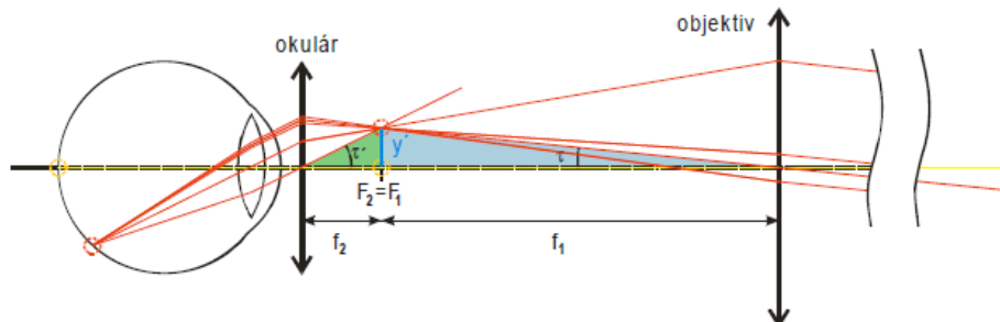
Obrázek 10.12: Schéma Keplerova dalekohledu k odvození zvětšení dalekohledu. Autor M. Krynický. Převzato z www.realisticky.cz .
