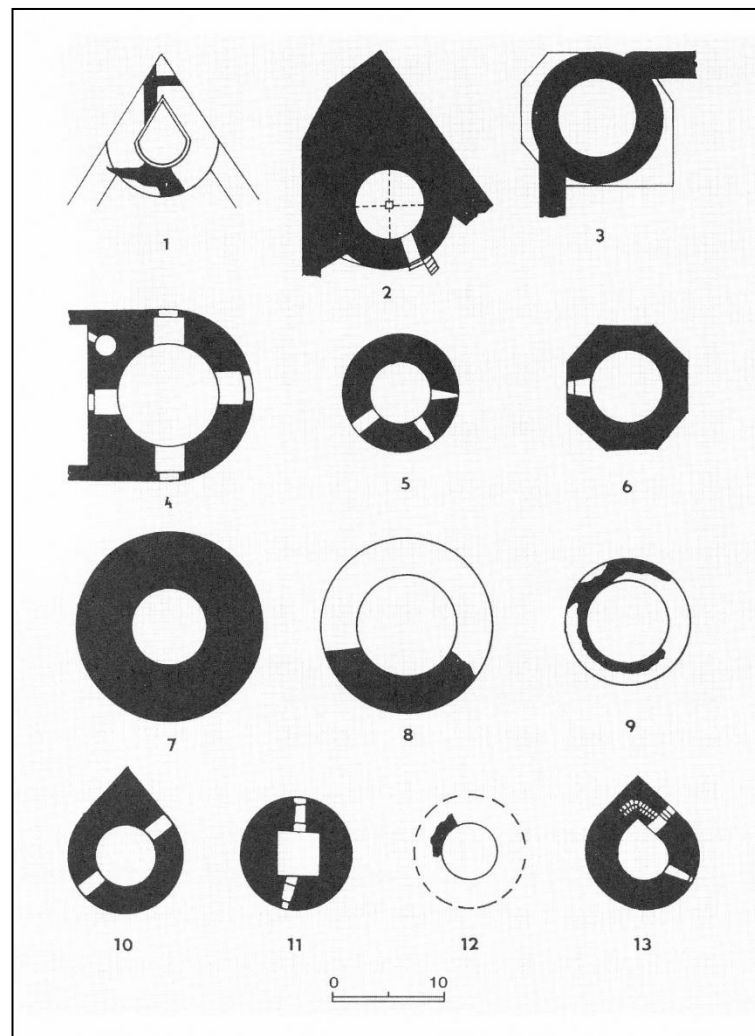
Hrady s obytnou věží – donjonového typu
