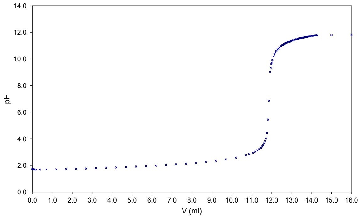
Obr.1 Titrační křivka HCl
