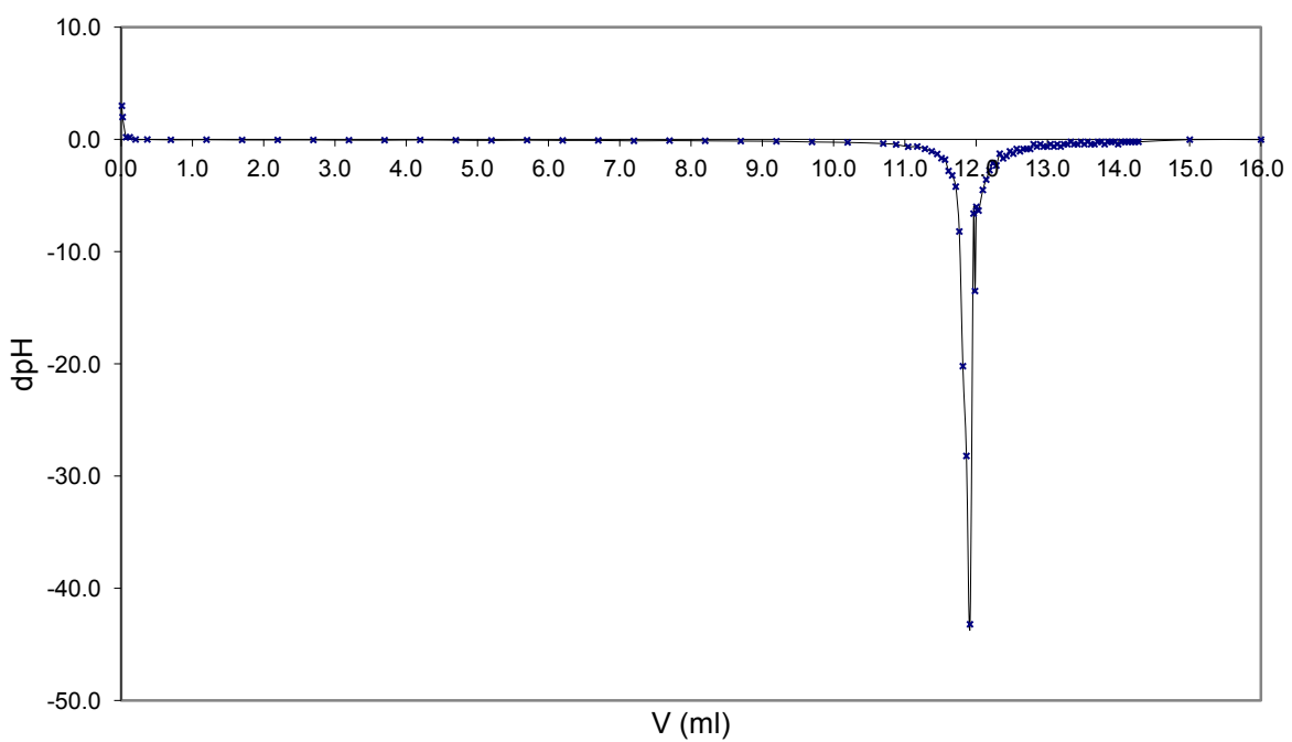
Obr.2 Derivační křivka HCl
