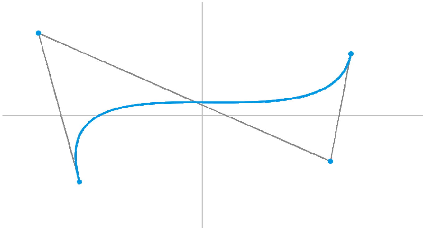
Obr. 1: Znáznění Bézierovy křivky
