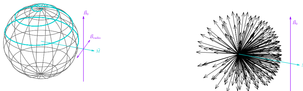
Obrázek 14.4: Vlevo znázornění pohybu vektoru magnetizace (jako azurová dráha na povrchu koule o poloměru |\vec{M}| ) v přítomnosti oscilujícího magnetického pole radiové vlny. Vpravo distribuce magnetických momentů jader po sklopení vektoru magnetizace do směru kolmého na \vec{B}_0 .
