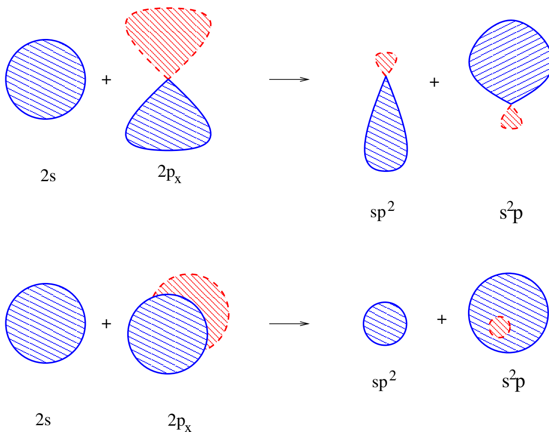
Obrázek 15.14: Orbitaly s 2 p
