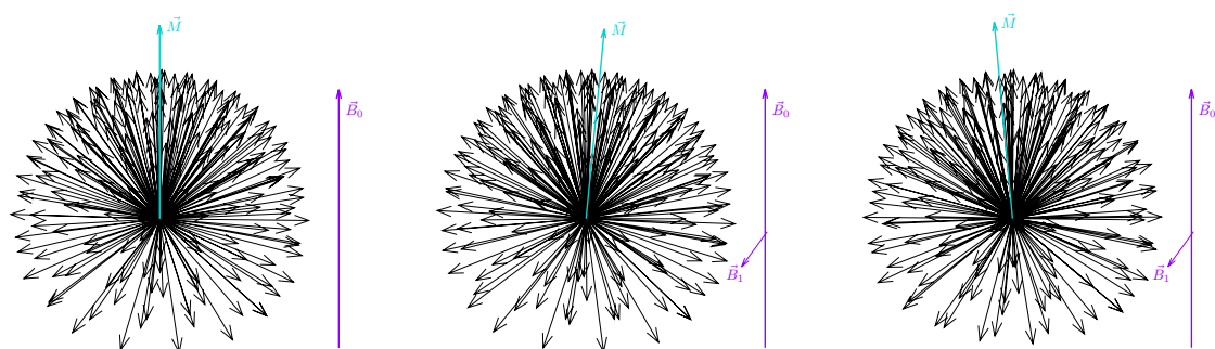
Obrázek 14.3: Vlevo je ukázána distribuce magnetických momentů jader ve vnějším magnetickém poli o indukci \vec{B}_0 (fialová šipka). Celkový magnetický moment je znázorněn jako azurová šipka. Uprostřed je ukázána distribuce magnetických momentů odpovídající magnetizaci (azurová šipka) vychýlené mírně doprava dalším magnetickým polem o indukci \vec{B}_1 (tenká fialová šipka), které otáčí magnetické momenty po směru hodinových ručiček. Vpravo je ukázána tatáž distribuce otočená o polovinu kruhu v důsledku precese kolem \vec{B}_0 . Slabší pole o indukci \vec{B}_1 , otáčející magnetické momenty po směru hodinových ručiček, v tento okamžik vrací vektor magnetizace (azurovou šipku) zpět do svislého směru.
