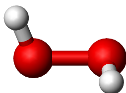
Obrázek 1.5: Molekula peroxidu vodíku.
