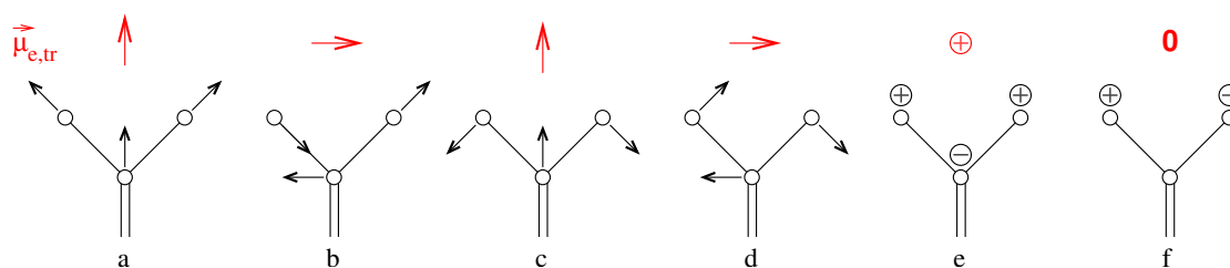
Obrázek 11.11: Vibrace tříatomové molekuly: a, symetrická valenční (in-phase stretching), b, asymetrická valenční (out-of-phase stretching), c, nůžková (in-plane in-phase bending), d, kývavá (in-plane out-of-phase bending), e, rotující (out-of-plane in-phase bending), f, twistová (out-of-plane out-of-phase bending). Na obrázku jsou vibrace v rovině papíru znázorněny šipkami, vibrace nad rovinu papíru \oplus a vibrace pod rovinu papíru \ominus . Červeně je vyznačen směr elektrického tranzitního momentu jednotlivých vibrací.
