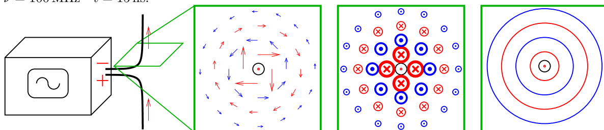
Obrázek 11.1: Ilustrace vzniku radiové vlny. Zdroj střídavého napětí mění polaritu s frekvencí \nu = 100 \text{ MHz} , jednotlivé obrázky ukazují elektromagnetické pole v intervalech 5 ns po zapnutí zdroje. V zelených rámečcích jsou (zprava doleva) nakresleny vektory \vec{B} , \vec{E} a hřebeny vzniklé kruhové vlny. Směr vzhůru (na levém náčrtku) kolmo k zelené rovině je znázorněn tečkou, směr dolů křížkem. Směr pohybu elektronů v kolmých řezech je znázorněn tečkou nebo křížkem uprostřed zeleného rámečku.
