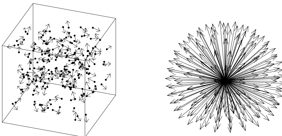
Obrázek 14.2: Vlevo zjednodušený obrázek vzorku proteinu studovaného pomocí NMR. Molekuly proteinu jsou znázorněny jako tečky. Pro každou molekulu je znázorněn jeden magnetický moment jako šipka. Vpravo znázornění orientací magnetických momentů v nepřítomnosti vnějšího magnetického pole. Počátky všech šipek z obrázku vlevo jsou umístěny do stejného bodu. Obrázek ukazuje, že magnetické momenty (šipky) míří se stejnou pravděpodobností do všech směrů.
