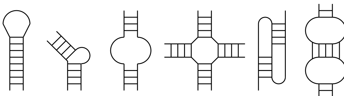
Obrázek 3.10: Příklady strukturních motivů nukleových kyselin. Zleva vláseňková smyčka ( hairpin loops ), zlom s včleněným nepárováným nukleotidem bulge , internal loop , four-way junction , pseudouzle pseudoknot , kissing hairpin .
