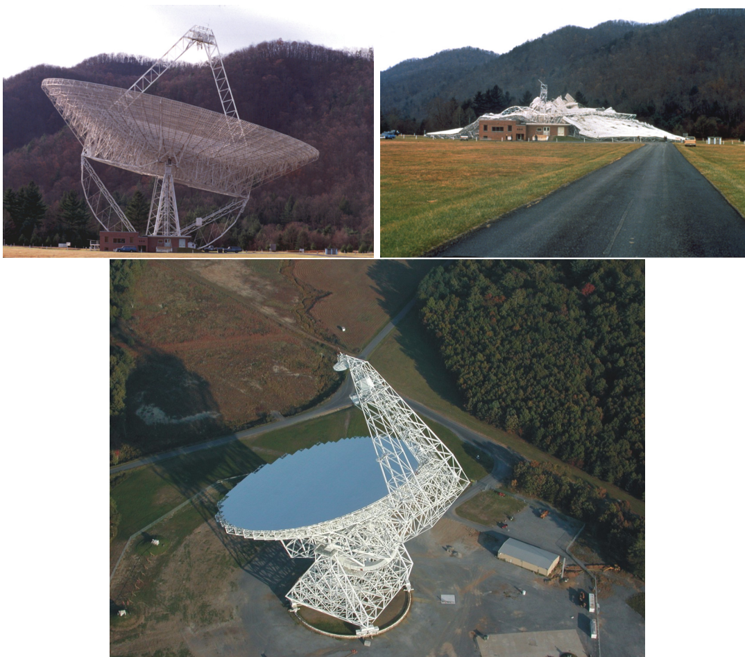
Obrázek 11.4: Nahoře: Původní velký radioteleskop v NRAO, Green Bank, 15. listopadu 1988 a vpravo následující den, po zhroucení. Dole: Zničený radioteleskop nahradil nový přístroj – Robert C. Byrd Green Bank Telescope. Foto: Richard Porcas, NRAO.
