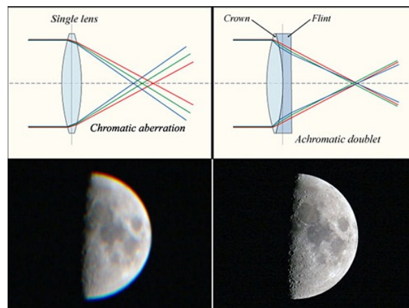
Obrázek 10.15: Levný dalekohled s jednoduchou čočkou vytváří rozmazaný obraz s okrajem s falešnými barvami (vlevo). Galileoscope (vpravo) představuje kvalitnější achromát tvořený dvojitou čočkou. Ohnisko je společné pro modré a červené světlo, ohnisko zeleného světla je lehce posunuté. Zdroje: Schémata R. Caniatti/Wikipedia, snímky Měsíce R. Fienberg.
