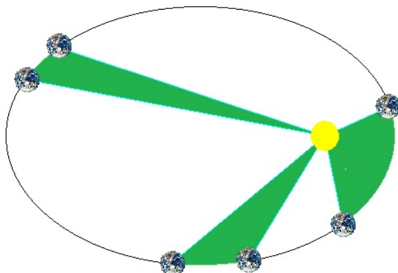
Obrázek 12.38: Druhý Keplerův zákon. Převzato z http://astronomia.zcu.cz .
