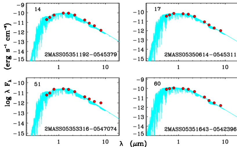
Obrázek 9.3: Rozložení energie ve spektru (SED; Spectral energy distribution) čtyř hvězd z katalogu 2MASS. Červené body představují výsledky fotometrických měření, světle modře je zobrazeno uměle spočtené spektrum hvězd, které nejlépe odpovídá fotometrickým pozorováním. Zdroj: Frasca et al. (2009).
