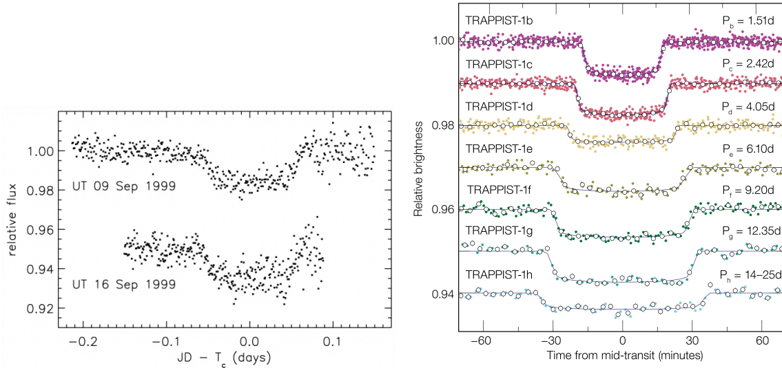
Obrázek 13.10: Vlevo: První zaznamenané tranzity exoplanety HD 209458 b. Zdroj: Charbonneau et al. (2000). Vpravo: Transity planet v unikátní soustavě TRAPPIST-1. Zdroj: https://www.eso.org/public/news/eso1706/
