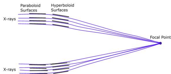
Obrázek 11.2: Schéma rentgenového dalekohledu Wolterovy konstrukce. Rentgenové záření je zde soustředěno pomocí několika sousých rotačních parabolických a hyperbolických ploch vložených do sebe. Převzato z http://ixo.gsfc.nasa.gov/images/science .
