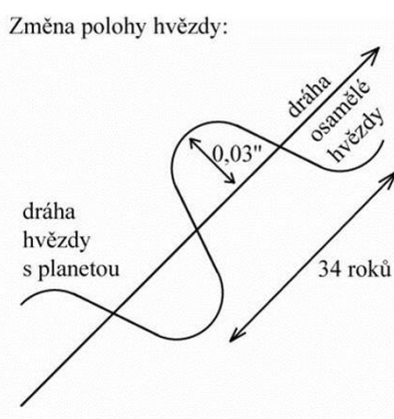
Obrázek 13.5: Možnosti astrometrické detekce exoplanet. Převzato z Pokorný (2006).
