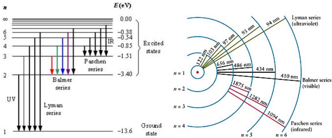
Obrázek 7.13: Schématické znázornění přeskoků elektronů mezi hladinami nejjednodušší atomové struktury (atomu vodíku). Vpravo jsou uvedeny vlnové délky vyzářených fotonů. Převzato z http://www.daviddarling.info/encyclopedia/H/hydrogen_spectrum.html .
