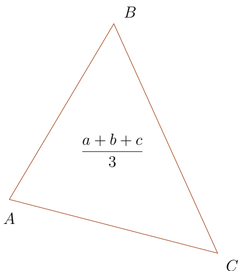
Obrázek 1: Trojúhelník s popisem
