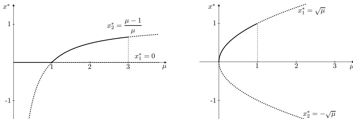
Obrázek 4.3: Rovnovážné body logistické rovnice (4.14) (vlevo) a rovnice (4.15) (vpravo) v závislosti na hodnotách parametru \mu . Asymptoticky stabilní rovnovážný bod je znázorněn plnou čarou, nestabilní tečkovanou čarou.
