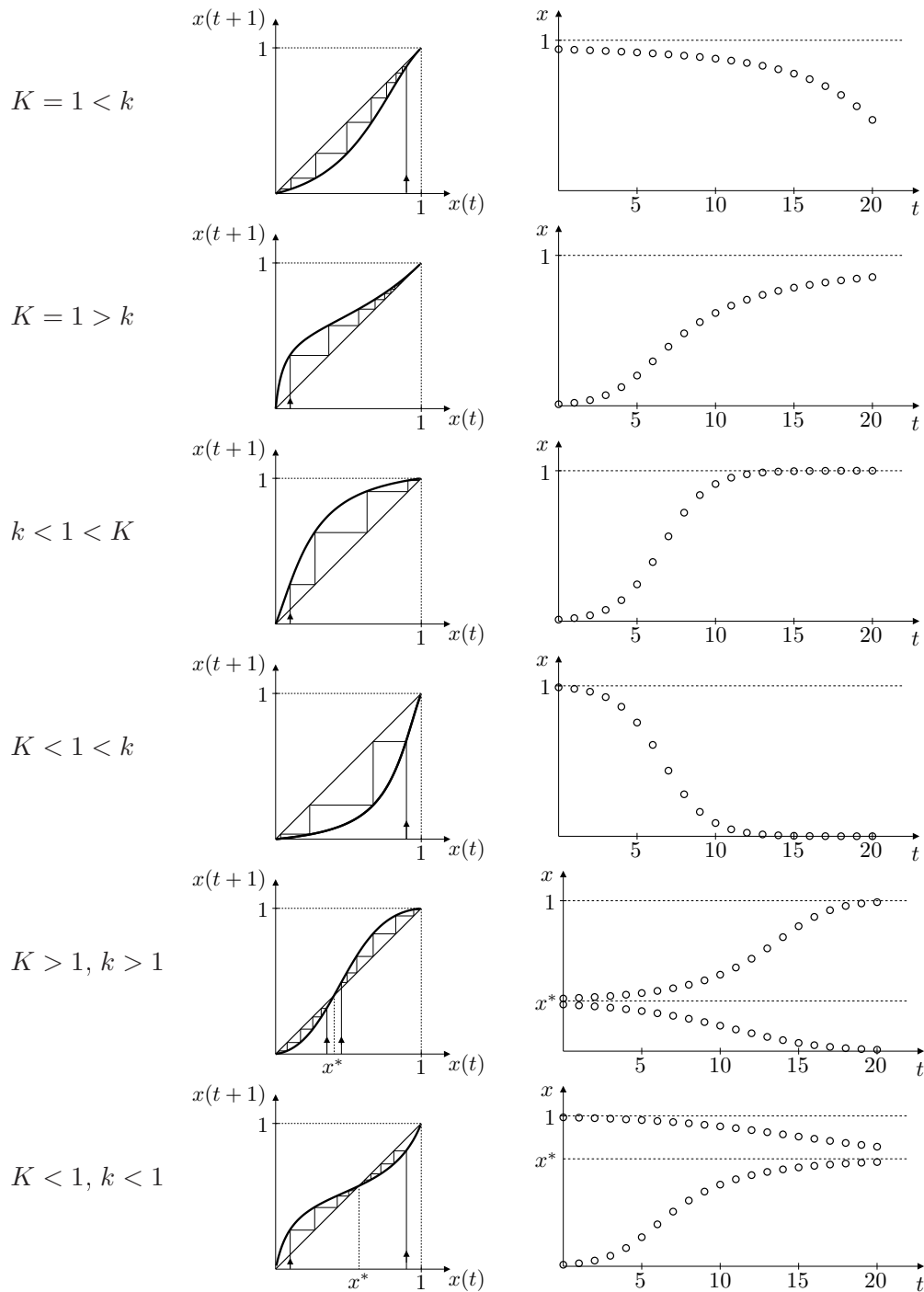
Obrázek 5.8: Grafické řešení rovnice (5.115) a jeho průběh pro různé hodnoty parametrů K , k . Tj. vývoj relativní frekvence alely A v populaci pro různé relativní reprodukční zdatnosti homozygotů vzhledem k heterozygotům.
