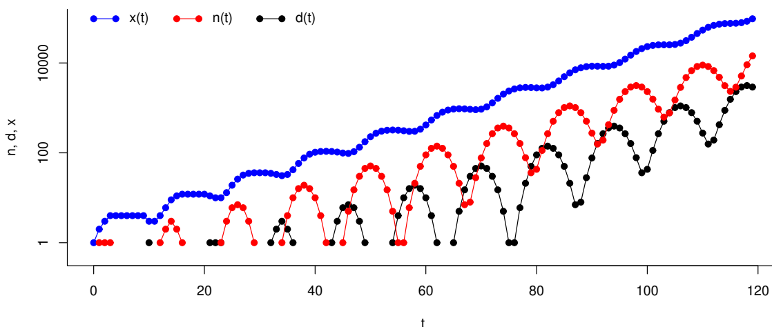
Obrázek 5.2: Model „rozmnožování lidského rodu“ (5.19). Na svislé ose je logaritmické měřítko. Symboly označují: x(t) — počet žijících párů v čase t , tj. 2t let od počátku, n(t) — počet narození v čase t , d(t) — počet úmrtí v čase t .
