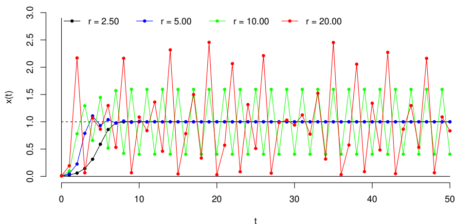
Obrázek 1.4: Řešení Rickerovy rovnice x(t+1) = x(t)r^{1-x(t)} s počáteční hodnotou x(0) = 0,01 pro několik hodnot parametru r . Pro r = 2,5 je řešením rostoucí posloupnost s limitou 1 (rovnovážná velikost populace), pro r = 5 řešení konverguje k hodnotě 1 s tlumenými oscilacemi, pro r = 10 řešení pro dostatečně velký čas t (zhruba od t = 10 ) pravidelně kolem hodnoty 1 kolísá, pro r = 20 již žádnou pravidelnost v chování řešení nelze vypozorovat.
