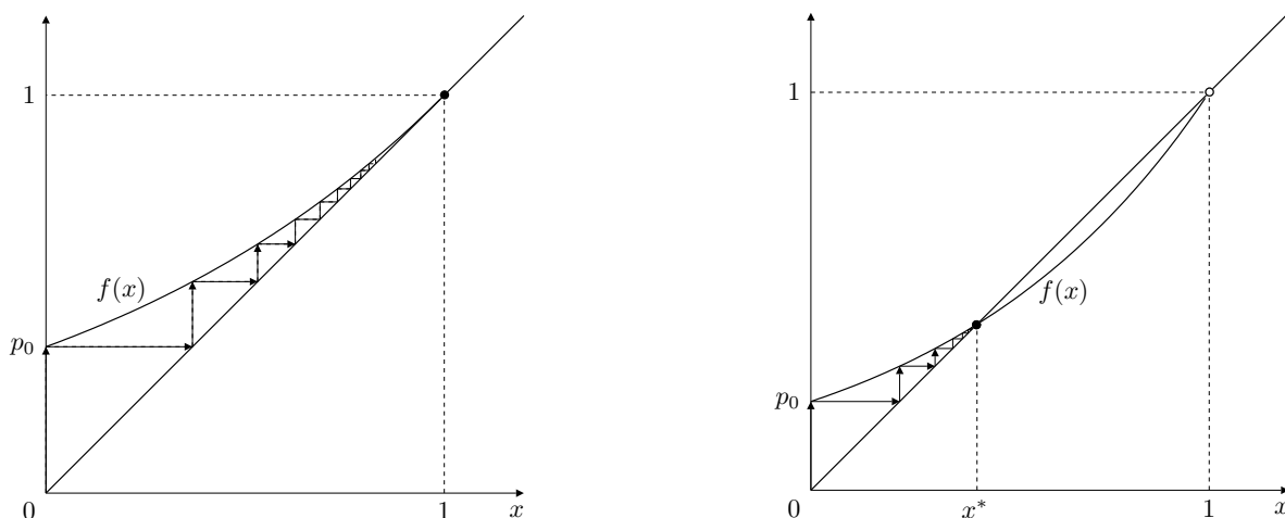
Obrázek 5.4: Grafické řešení počáteční úlohy (5.61), (5.56) v případě f'(1) \leq 1 (vlevo) a f'(1) > 1 (vpravo).
