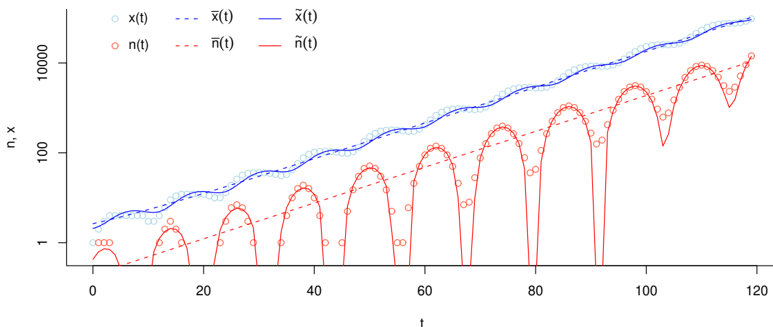
Obrázek 5.3: Upravený model „rozmnožování lidského rodu“ (5.20). Na svislé ose je logaritmické měřítko. Symboly označují: x(t) , n(t) — hodnoty počítané z rekurentních vztahů (5.20), \bar{x}(t) , \bar{n}(t) — první aproximace řešení (5.22) využívající pouze dominantní charakteristický kořen \lambda_1 (trend), \tilde{x}(t) , \tilde{n}(t) — druhá aproximace řešení (5.24) využívající charakteristické kořeny \lambda_{2,3} s druhým největším modulem. Při výpočtu byly použity hodnoty \alpha \doteq 0,1947 , \bar{x}_0 \doteq 2,6515 , \beta \doteq 0,2319 , \gamma \doteq 0,3528 , \tilde{x}_0 \doteq 2,0736 .
