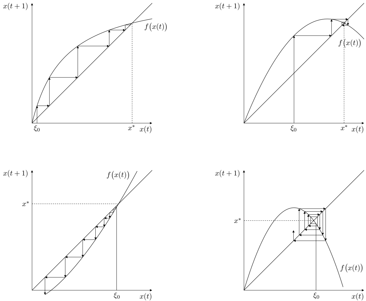
Obrázek 4.2: Grafické řešení autonomní rovnice (4.7). Vlevo „schodový diagram“, vpravo „pavučinový diagram“, nahore stabilní (přitahující) pevný (rovnovážný) bod zobrazení f , dole nestabilní (odpuzující).
