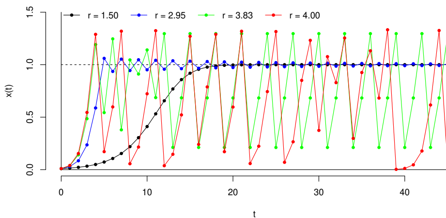
Obrázek 1.2: Řešení logistické rovnice x(t+1) = x(t)(r - (r-1)x(t)) s počáteční hodnotou x(0) = 0,01 pro několik hodnot parametru r . Pro r = 1,5 je řešením rostoucí posloupnost s limitou 1 (rovnovážná velikost populace), pro r = 2,95 řešení konverguje k hodnotě 1 s tlumenými oscilacemi, pro r = 3,83 řešení pro dostatečně velké hodnoty času t (zhruba od t = 15 ) skoro pravidelně osciluje kolem hodnoty 1 s periodou 3, pro r = 4 nelze žádnou pravidelnost řešení vysledovat.
