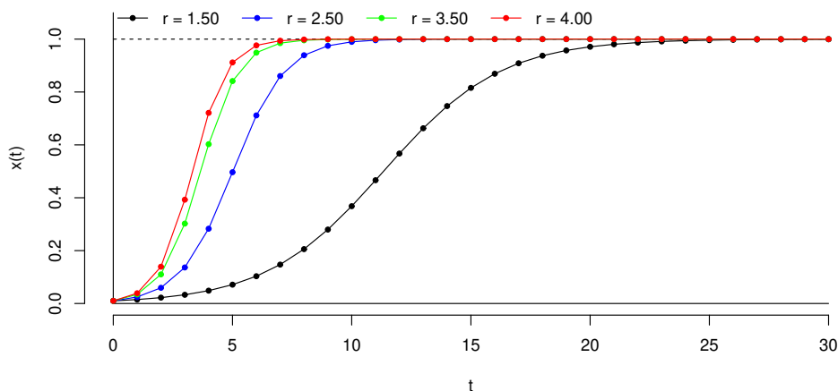
Obrázek 1.3: Řešení Bevertonovy-Holtovy rovnice x(t+1) = x(t) \frac{r}{1 + (r-1)x(t)} s počáteční hodnotou x(0) = 0,01 pro několik hodnot parametru r . Ve všech případech je řešením rostoucí posloupnost s limitou 1 (tj. hodnotou rovnovážné velikosti populace).
