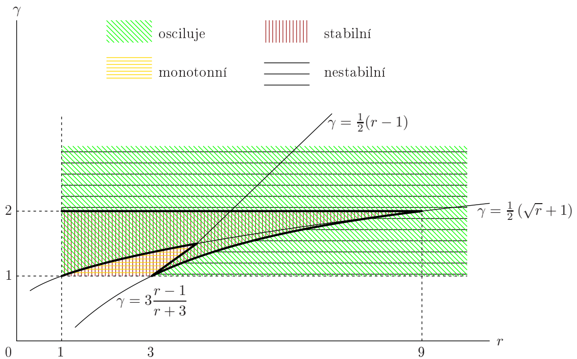
Obrázek 5.6: Závislost kvalitativních vlastností řešení systému (5.94) (modelu dravec-kořist J. Maynarda Smithe) v okolí vnitřního stacionárního bodu (koexistenční rovnováhy) na hodnotách růstového koeficientu kořisti r a „efektivity predace“ \gamma .
