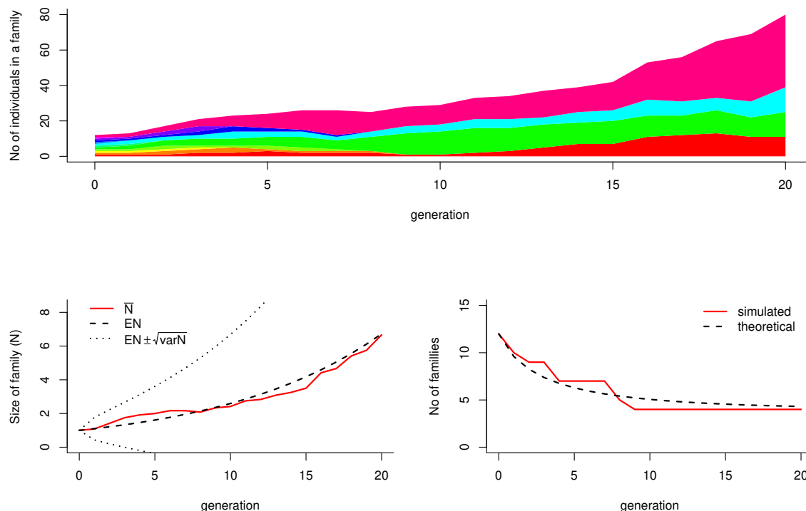
Obrázek 5.5: Ilustrace výsledků Příkladu 3. Simulace vývoje dvaceti generací populace, kterou založilo N(0) = 12 rodin. Přitom ve všech rodinách jsou stejné pravděpodobnosti, že žádný syn se nedožije dospělosti p_0 = \frac{1}{5} , že se právě jeden dožije dospělosti p_1 = \frac{1}{2} a že se právě dva synové dožijí dospělosti p_2 = \frac{3}{10} . Nahoře: Počet mužských příslušníků populace v jednotlivých generacích; každé rodině odpovídá jedna barva. Po dvaceti generacích přežívají čtyři rodiny. Dole vlevo: Vývoj velikosti N(t) jedné rodiny. Černá čárkovaná čára vyjadřuje očekávanou velikost rodiny y(t) = EN(t) = \left(\frac{11}{10}\right)^t , černá tečkovaná čára vyjadřuje rozpětí směrodatné odchylky velikosti rodiny v jednotlivých generacích kolem její střední hodnoty y(t) \pm \sqrt{z(t)} . Červená plná čára je průměr ze simulovaných velikostí rodin. Dole vpravo: Počet rodin v populaci v jednotlivých generacích. Červená čára je počet simulovaných rodin s nenulovou velikostí (přežívajících), černá čárkovaná čára vyjadřuje teoretický počet x(t)N(t) přežívajících rodin.
