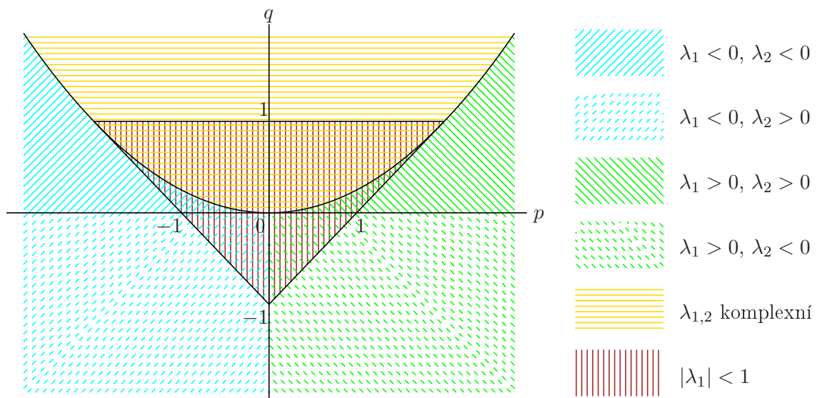
Obrázek 3.2: Závislost vlastních čísel matice Q příslušné k systému (3.50) na hodnotách p = \text{tr } Q a q = \det Q . Parabola má rovnici q = \frac{1}{4}p^2 , vlastní čísla jsou označena tak, že |\lambda_1| \geq |\lambda_2| .
