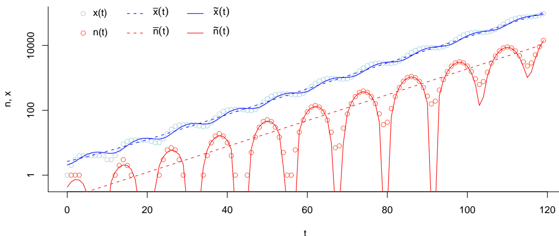
Obrázek 5.3: Upravený model „rozmožování lidského rodu“ (5.20). Na svislé ose je logaritmické měřítko. Symboly označují: x(t) , n(t) — hodnoty počítané z rekurentních vztahů (5.20), \bar{x}(t) , \bar{n}(t) — první aproximace řešení (5.22) využívající pouze dominantní charakteristický kořen \lambda_1 (trend), \tilde{x}(t) , \tilde{n}(t) — druhá aproximace řešení (5.24) využívající charakteristické kořeny \lambda_{2,3} s druhým největším modulem. Při výpočtu byly použity hodnoty \alpha \doteq 0,1947 , \bar{x}_0 \doteq 2,6515 , \beta \doteq 0,2319 , \gamma \doteq 0,3528 , \tilde{x}_0 \doteq 2,0736 .
