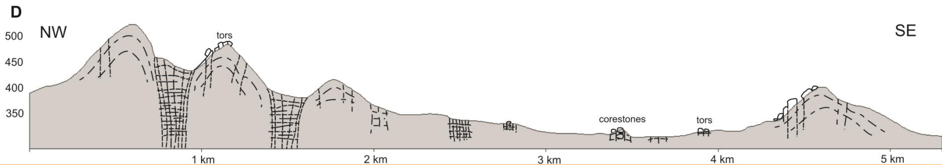
Etchplén - bazální zvětrávací plocha
