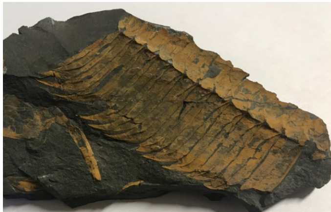
Trupový štít trilobita. Výuk. sb.
