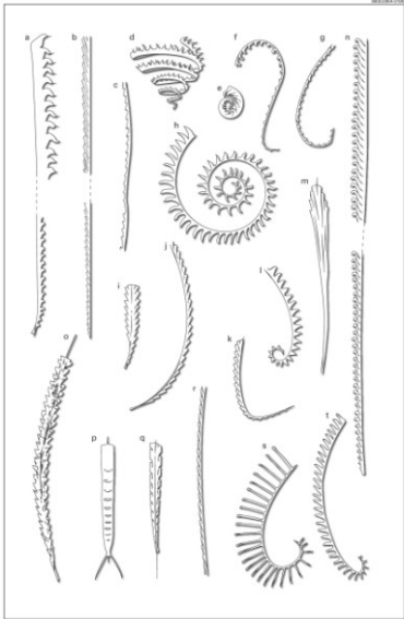
Graptoliti v břidlici. Výuk. sb.
