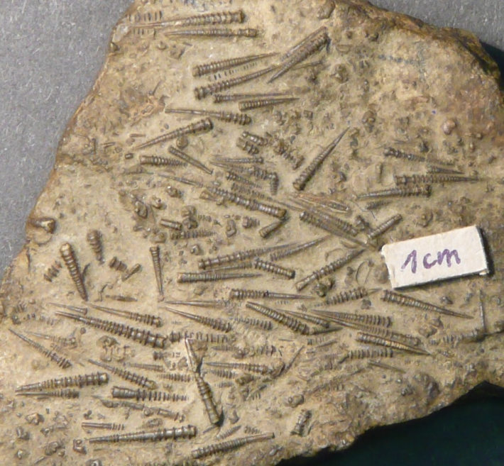
Tentakuliti ve vápenci.
